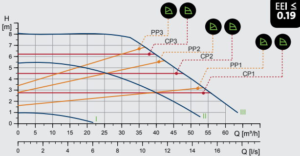
MAGNA1 100-80 F
