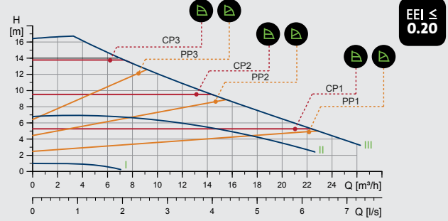
MAGNA1 40-180 F (N)
