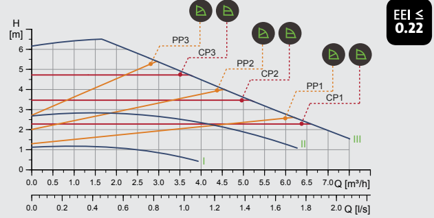
MAGNA1 25-60 (N)
