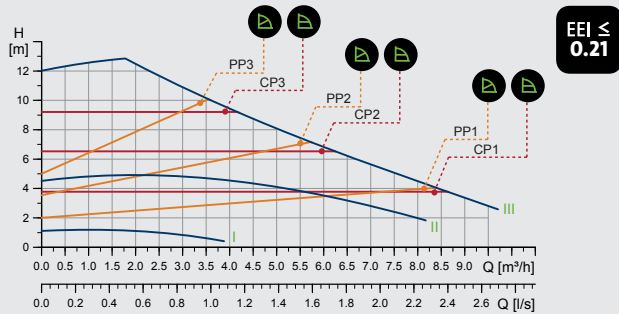
MAGNA1 25-120 (N)
