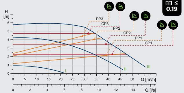
MAGNA1 100-60 F
