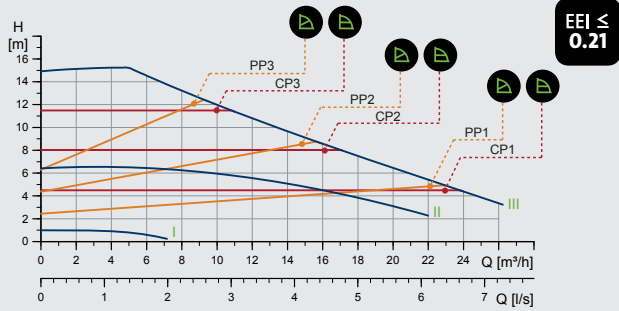
MAGNA1 40-150 F (N)
