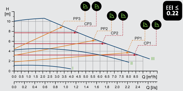
MAGNA1 25-100 (N)
